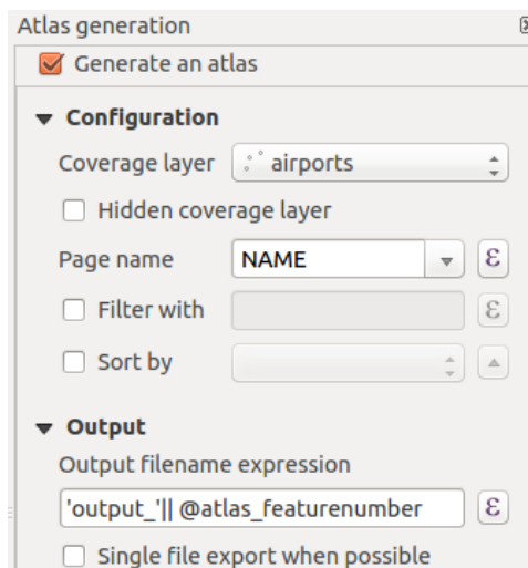
Рис. 17.60: Atlas Panel
