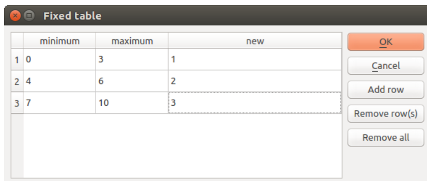
Рис. 22.15: Fixed Table
