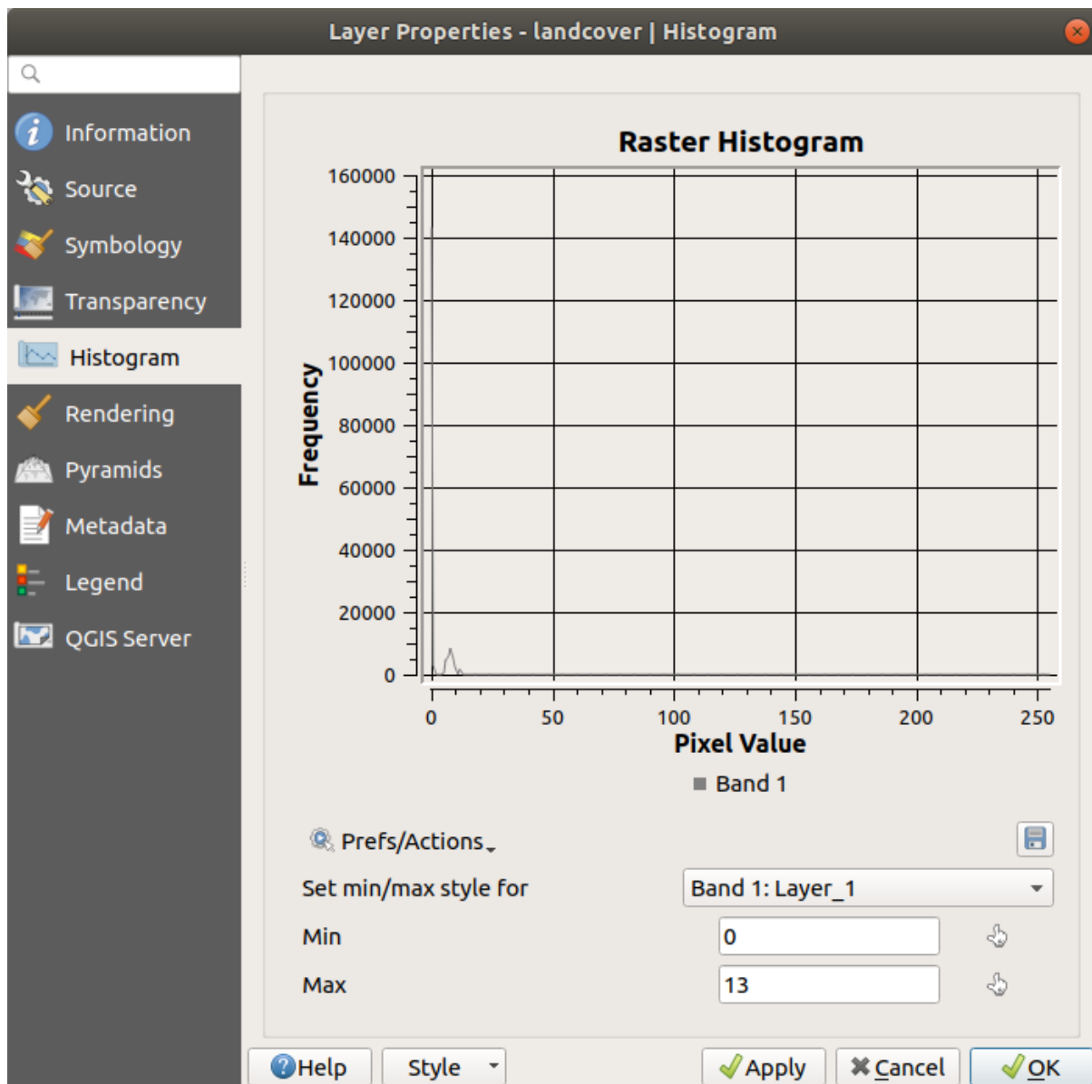
Рис. 15.10: Raster Histogram
