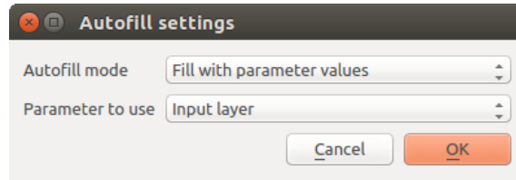
Рис. 22.31: Диалог автозаполнения
