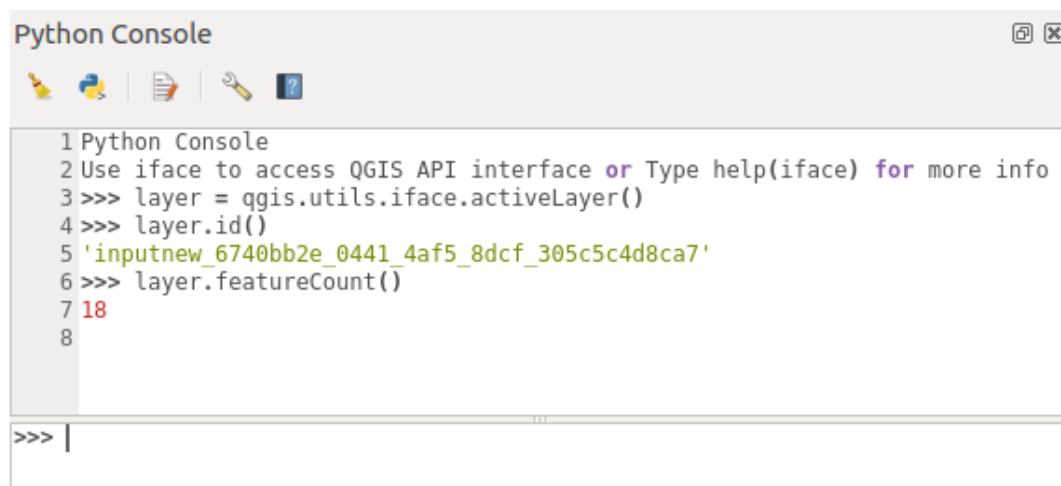
Abb. 1.1: QGIS Python Konsole
