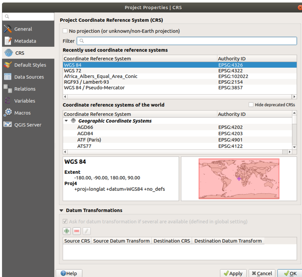
Obr. 10.2: Dialog vlastností projektu
