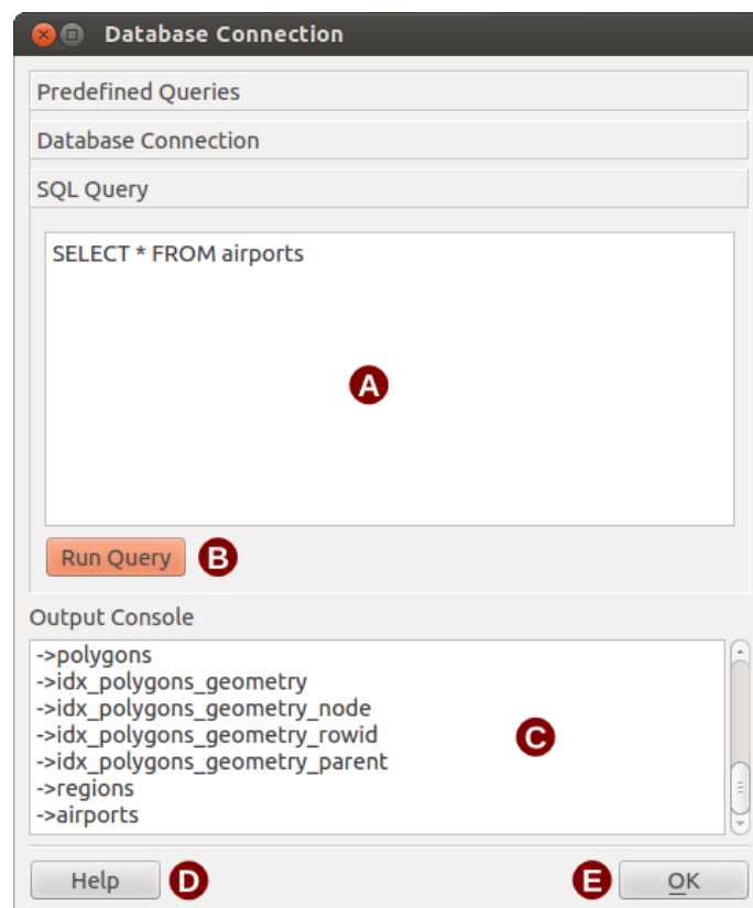
Рис. 19.14: Вкладка «SQL-запрос» расширения eVis
