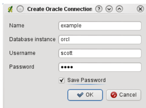
Рис. 19.26: Диалоговое окно «Создать соединение Oracle»
