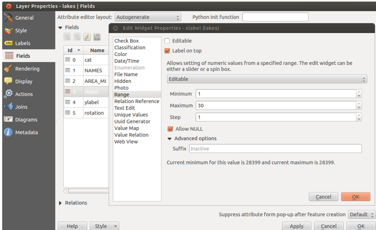
Рис. 12.28: Диалог выбора элемента редактирования поля 🐧
