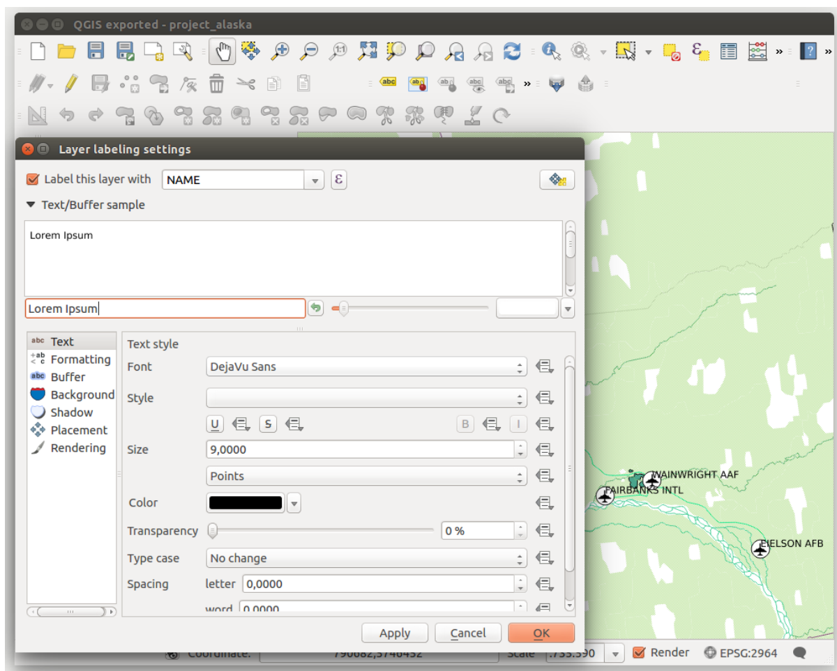
Рис. 12.22: Элегантные подписи для точечных векторных слоёв 🐧
