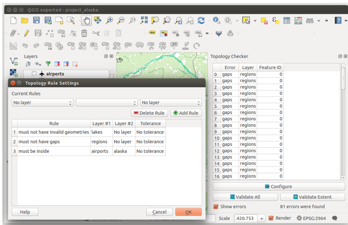
Рис. 19.33: Модуль «Проверка топологии»
