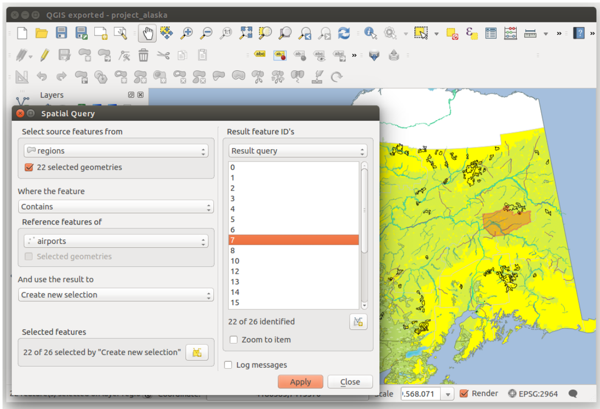
Рис. 19.31: Пространственный запрос — области с аэропортами 🐧
