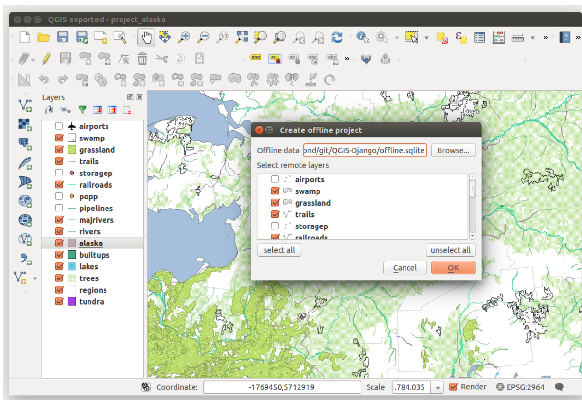
Рис. 19.25: Создание оффлайнового проекта из слоёв PostGIS или WFS
