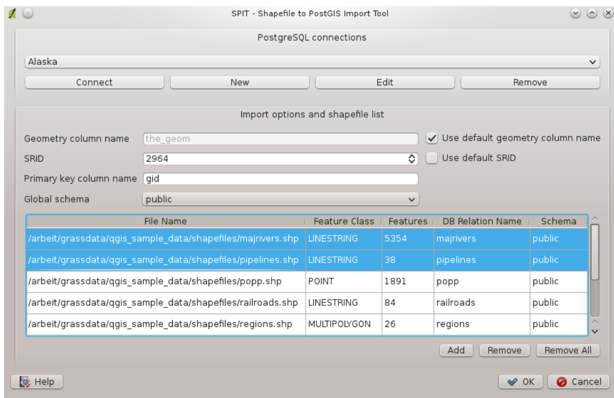
Рис. 19.32: Использование SPIT для импорта shape-файлов в PostGIS
