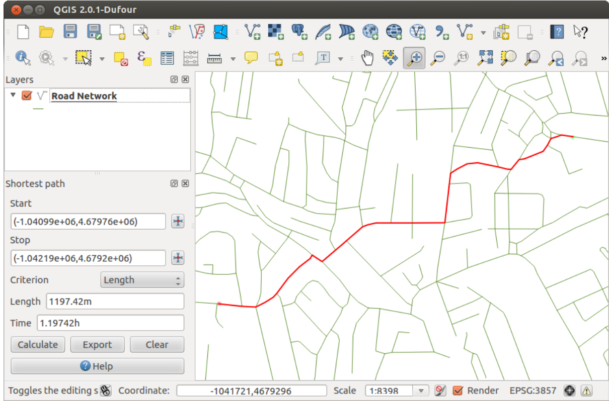
Figure 20.36: Yol Grafiği Eklentisi
