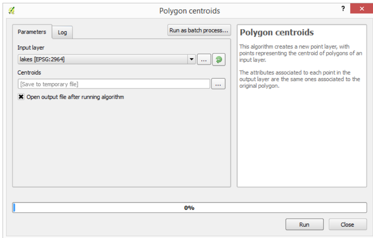
Рис. 18.8: Parameters Dialog
