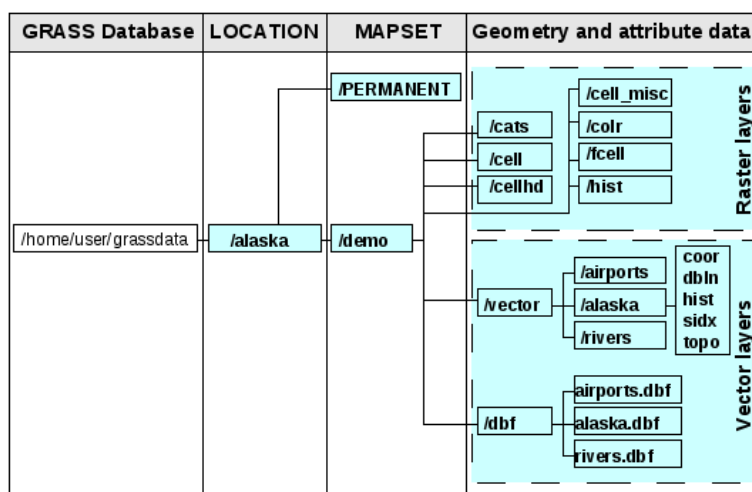
Рис. 17.1: Данные GRASS в районе «alaska»
