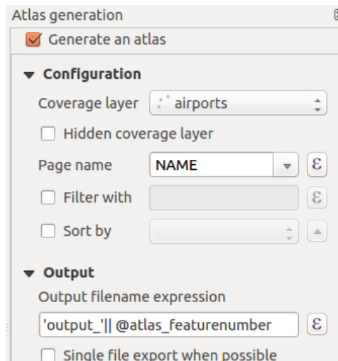
Рис. 19.50: Atlas generation tab
