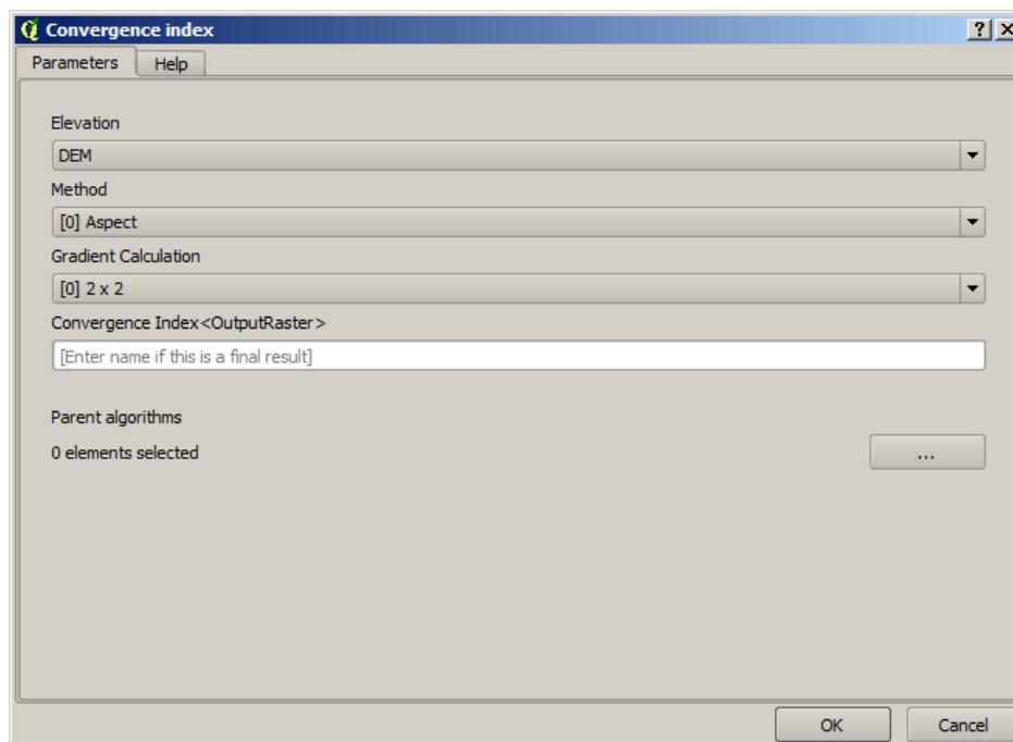
Рис. 18.21: Model Parameters
