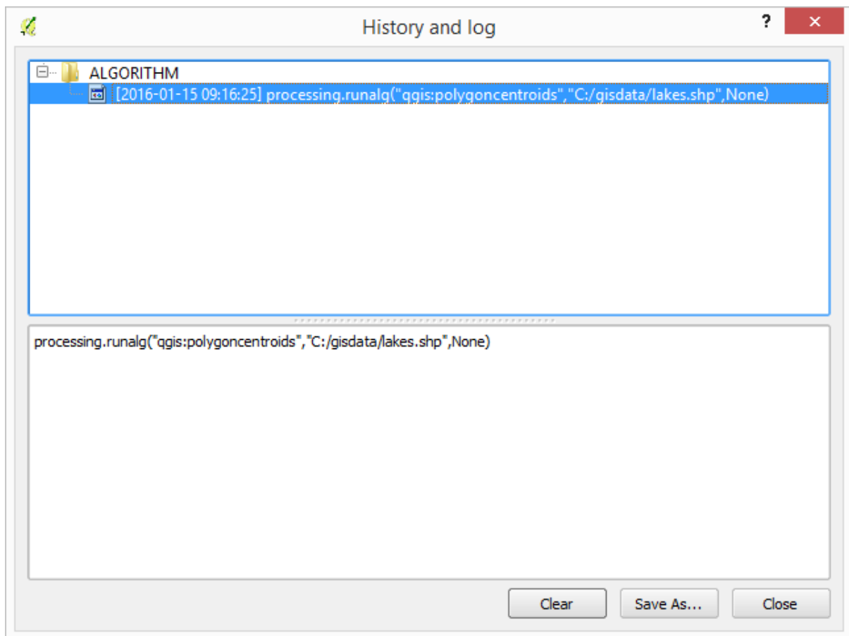
Figure 18.31: Histórico 🇧🇷
